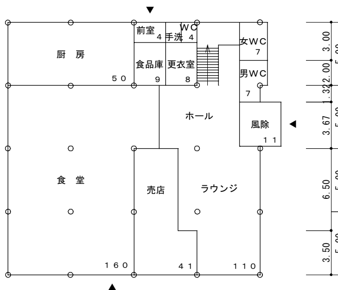
福利厚生施設 1階平面図 S = 1 / 300
