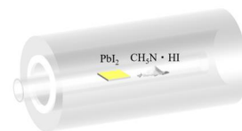
図3 アニール処理装置の概略図
