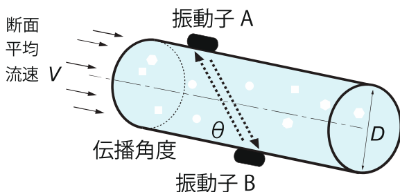
Fig. 1 計測原理
