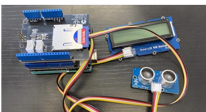
図-3 自作したArduino水位計
