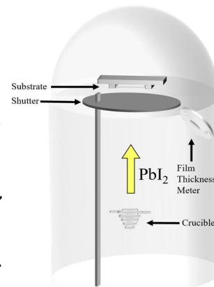
図2 真空蒸着装置の概略図
