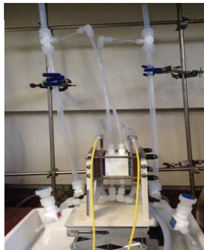
電気分解槽セル(試作)
