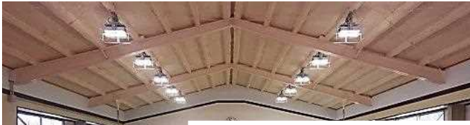
【武道場】 天井を撤去し、照明に落下防止ワイヤーを施しLED化。
