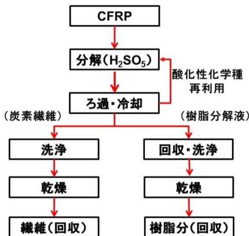
回収プロセス工程フロー
