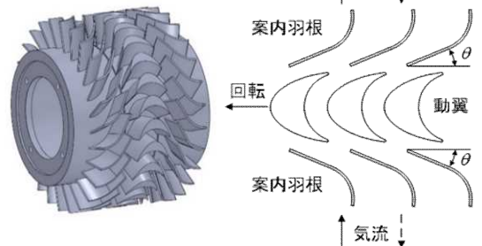
図3 往復流型衝動タービン
